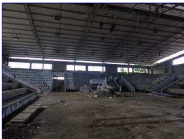
Vista interna del Gimnasio de Boxeo Alexis Arguello, a la izquierda se puede apreciar situación sin proyecto, en la fotografía de la derecha apreciar el inicio de ejecución de las obras con la limpieza general del sitio.
